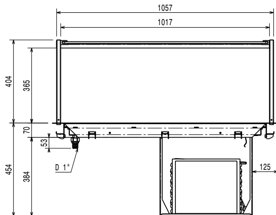
Front aanzicht
