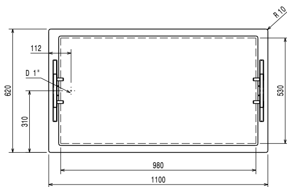
Boven aanzicht
